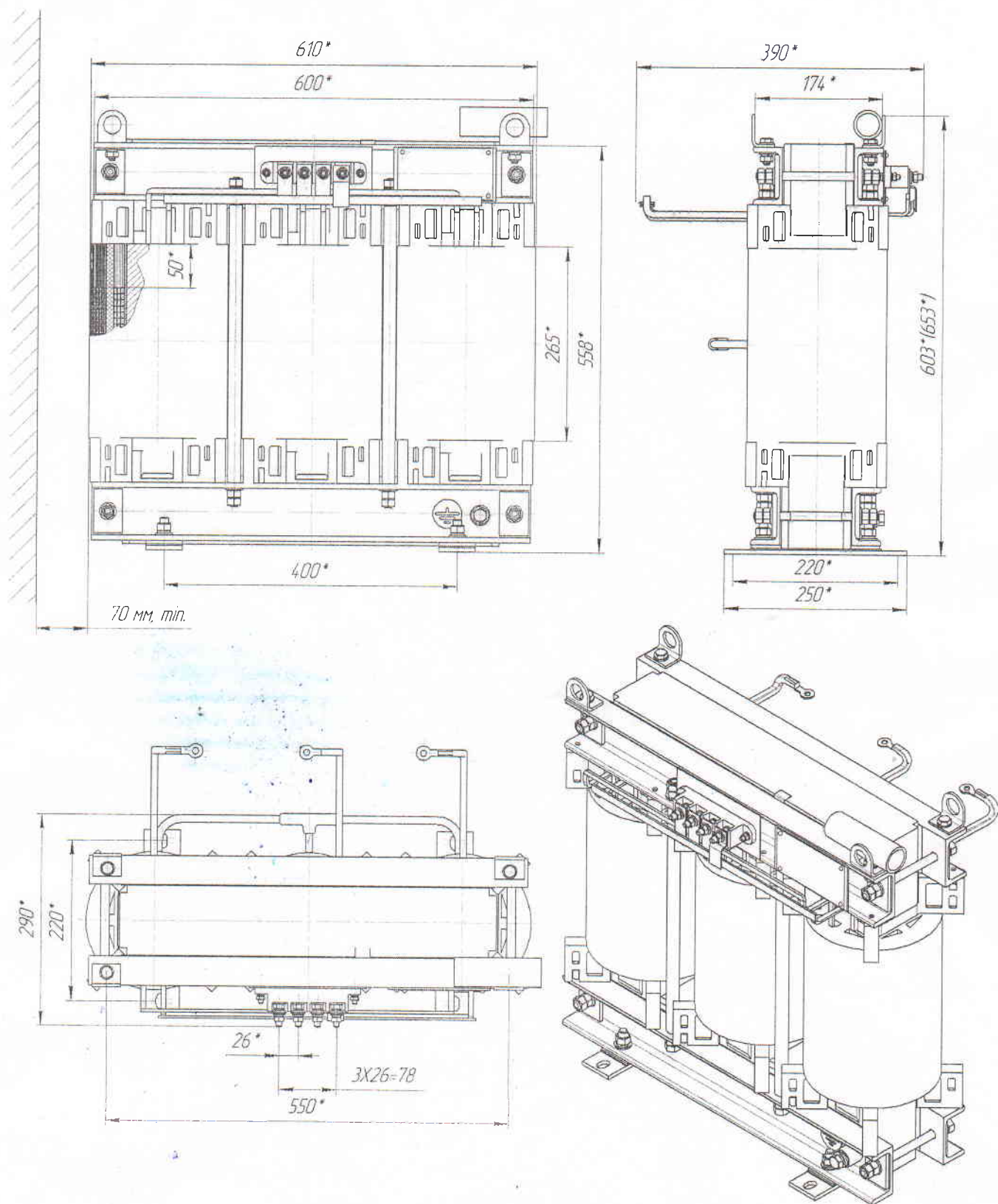
Рисунок 1 - Общий вид, габаритные, установочные и присоединительные размеры трансформатора типа ТСКС-16/10 – УЗ.
